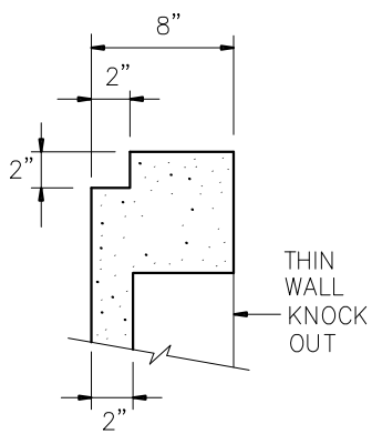
TYP. WALL DETAIL 72" X 72"
